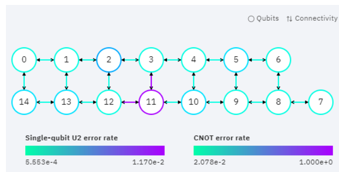
ภาพที่ 21 แสดงตำแหน่งและการเชื่อมโยงระหว่างคิวบิตบนเครื่องไอบีเอ็มเมลเบิร์น (Melbourne)
