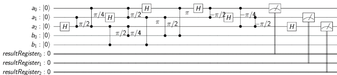
ภาพที่ 24 แสดงวงจรวกขนาด 2 คิวบิต ของ a และ b ซึ่ง a มีคิวบิตสำหรับตัวทดขนาด 1 คิวบิต
