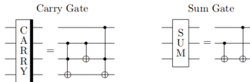
ภาพที่ 9 (ซ้าย) เกตแครี่ที่ประกอบขึ้นจากเกตซีซีนี้อยู่ (ขวา) เกตรวมที่ประกอบขึ้นจากเกตซีซีนี้อยู่ [2]
