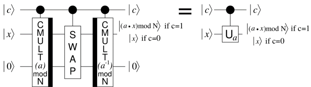
ภาพที่ 18 วงจรแลกเปลี่ยนเพื่อให้วงจรเป็นวงจรที่สามารถย้อนกลับได้ [4]
