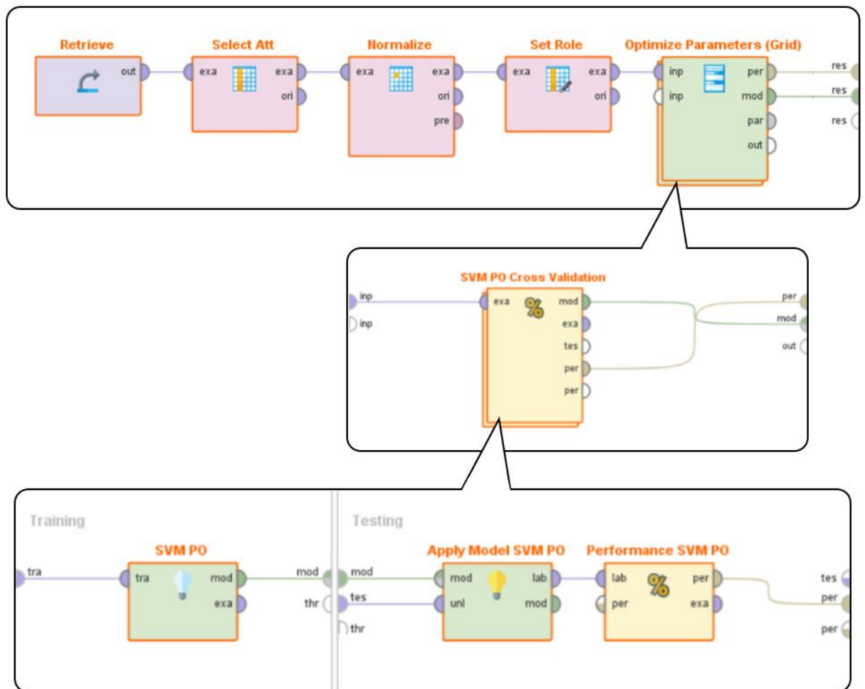
รูปที่ 33 ภาพแสดงแผนผังการทำงานภายในโปรแกรม RapidMiner Studio
