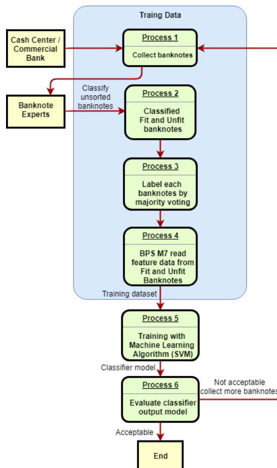
รูปที่ 29 ขั้นตอนการสร้าง Model แบ่งแยกธนบัตร
